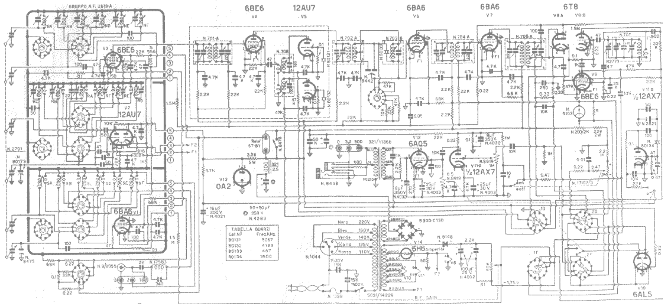
RICEVITORE PER ONDE CORTE G 209-R - GELOSO • SHORT WAVES RECEIVER G 209-R - GELOSO
